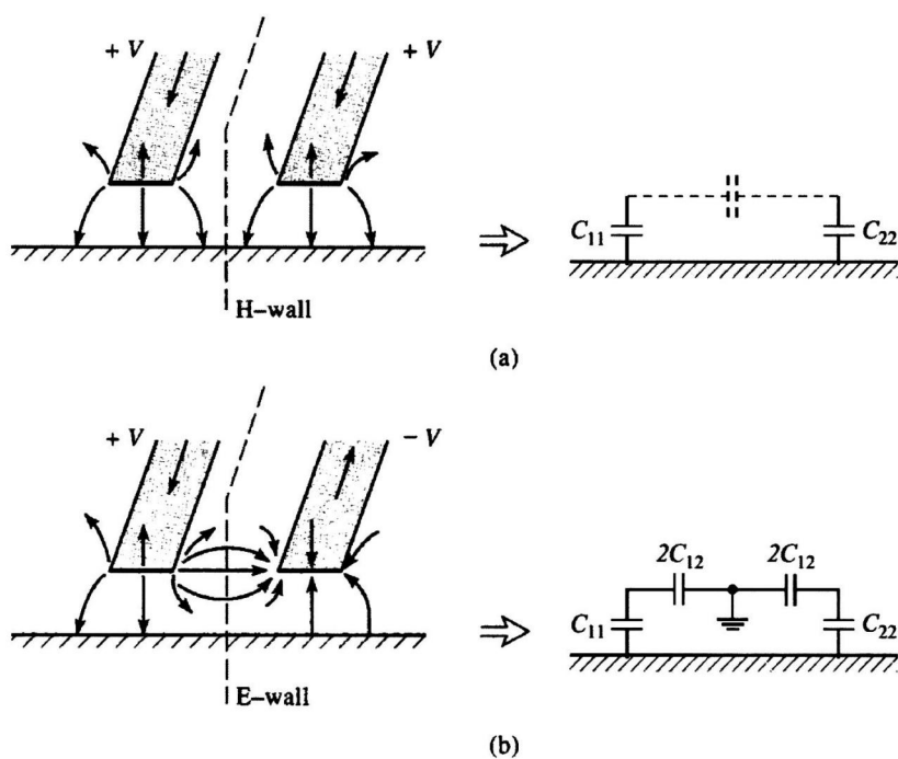
图 3.13 (a) 偶模激励 (b) 奇模激励 [48]
