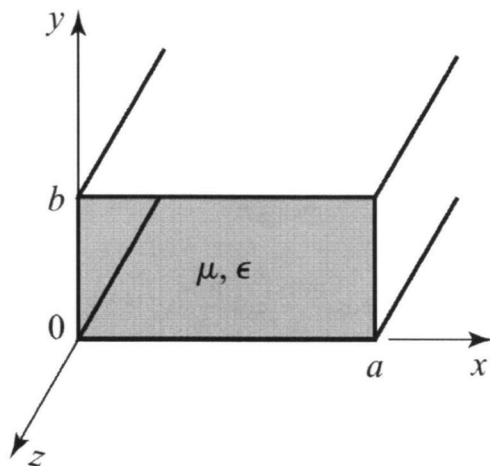
图 3.18 矩形波导结构
