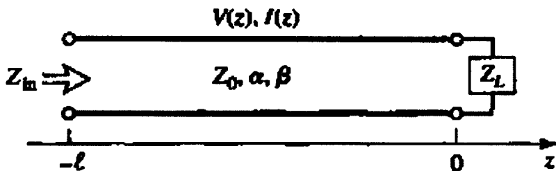
图 3.2 传输线模型
