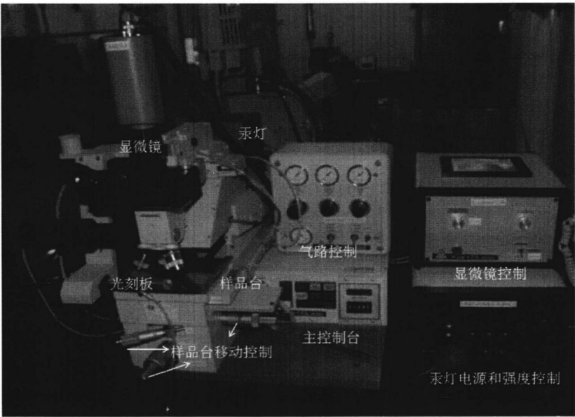
图 2.2 紫外光学曝光平台
