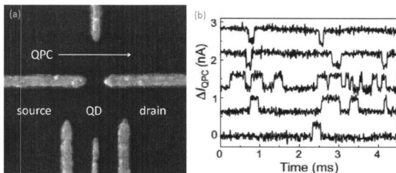
图 1.11 (a)QPC 结构 (b) 使用 QPC 测得的量子点中电子隧穿信号 [15]
