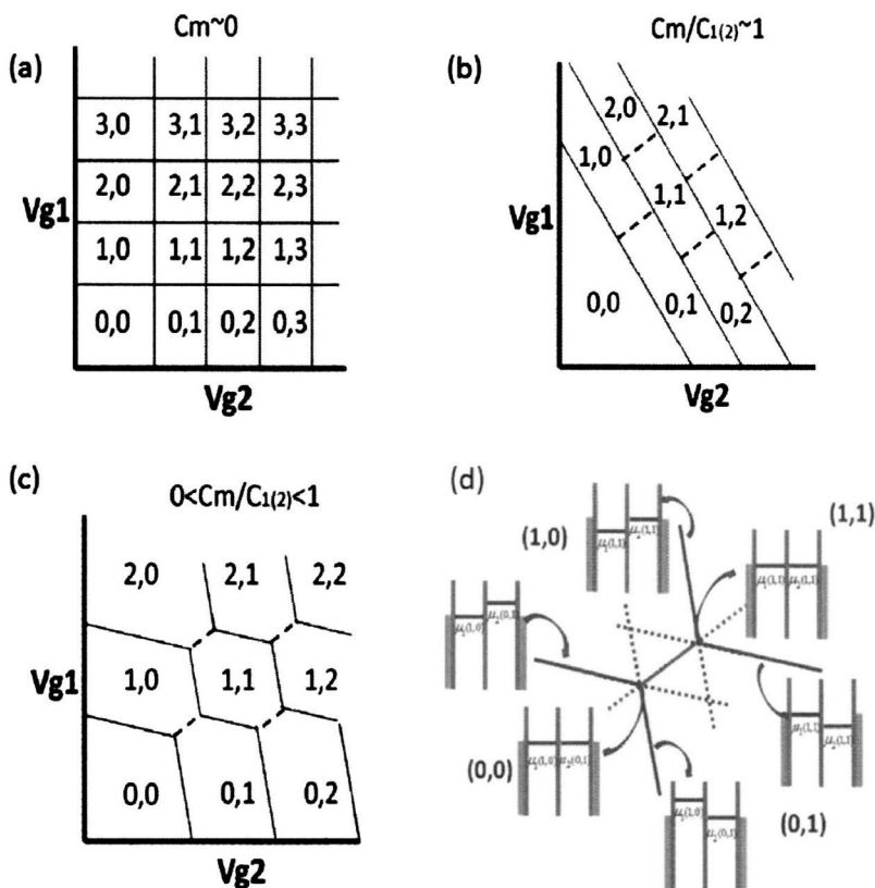
图 1.7 双量子点蜂窝相图 (a) 弱耦合 (b) 强耦合 (c) 中等耦合 (d) 量子点能级分布的变化
