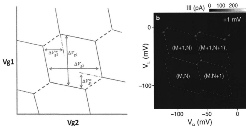
图 1.8 可从双量子点蜂窝相图中提取电容参数 [25]
