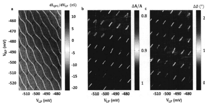
图 6.7 Graphene 双量子点电荷稳态相图 (a) 使用 QPC 调制测量 (b) 同样电压扫描区域谐振腔振幅变化信号 (c) 谐振腔相位变化信号
