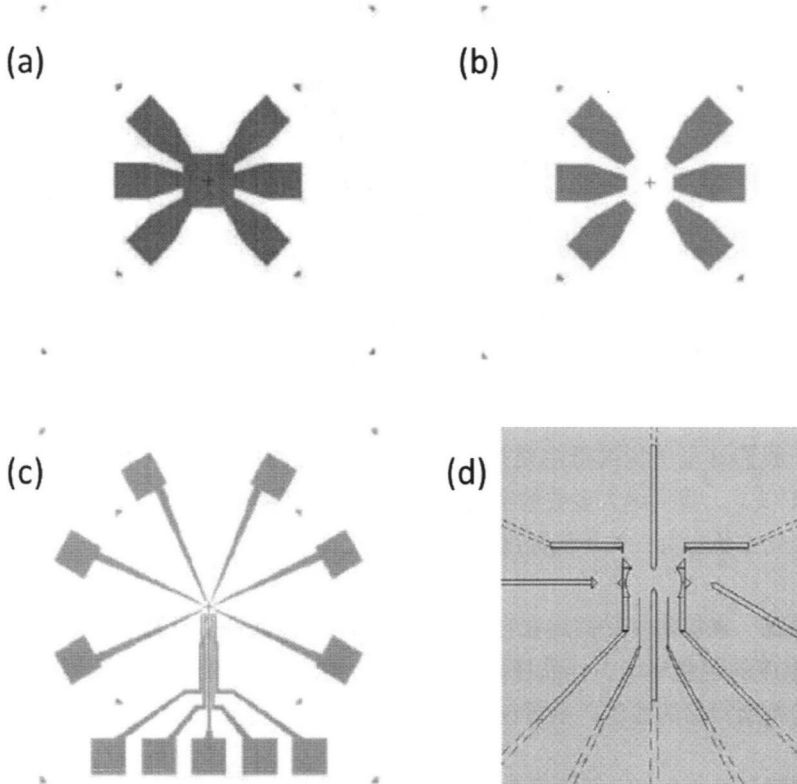
图 2.7 (a) mesa 光学曝光掩膜 (b) 欧姆电极光学曝光掩膜 (c) 表面大电极光学曝光掩膜 (d) 内部小电极 NPGS 设计图样
