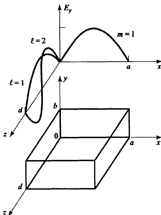
图 3.20 矩形谐振腔 [48]
